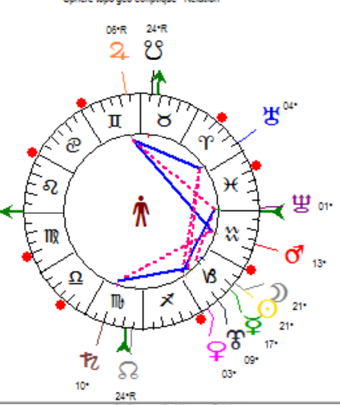
Sphère topo-géo-écliptique - Relation
