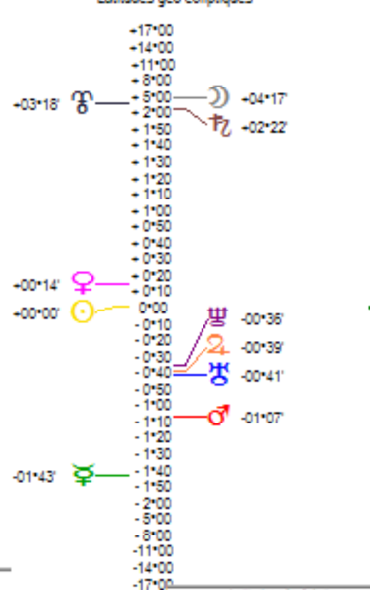
Latitudes géo-écliptiques
