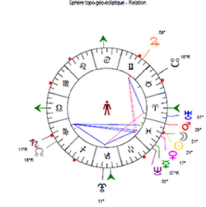
Sphère topo-géo-écliptique - Relation
