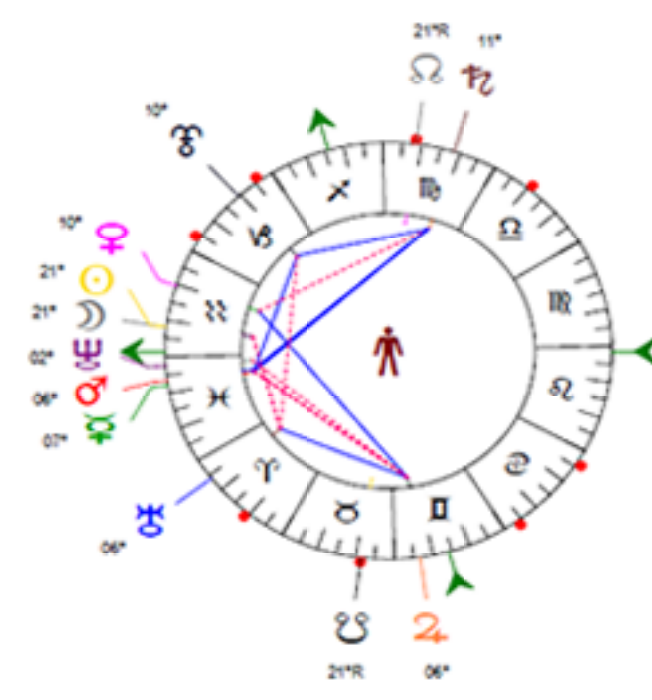
Sphère topo-géo-écliptique - Relation
