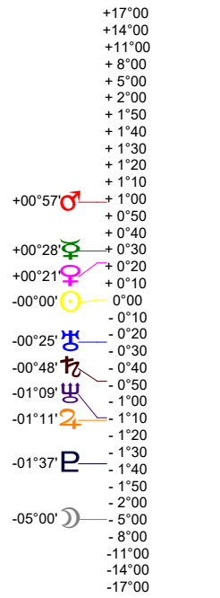
Latitudes géo-écliptiques
