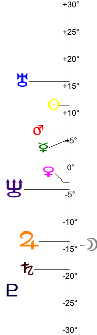
Déclinaisons
