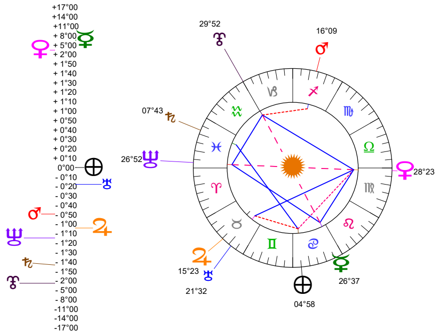
Latitudes héliocentriques
