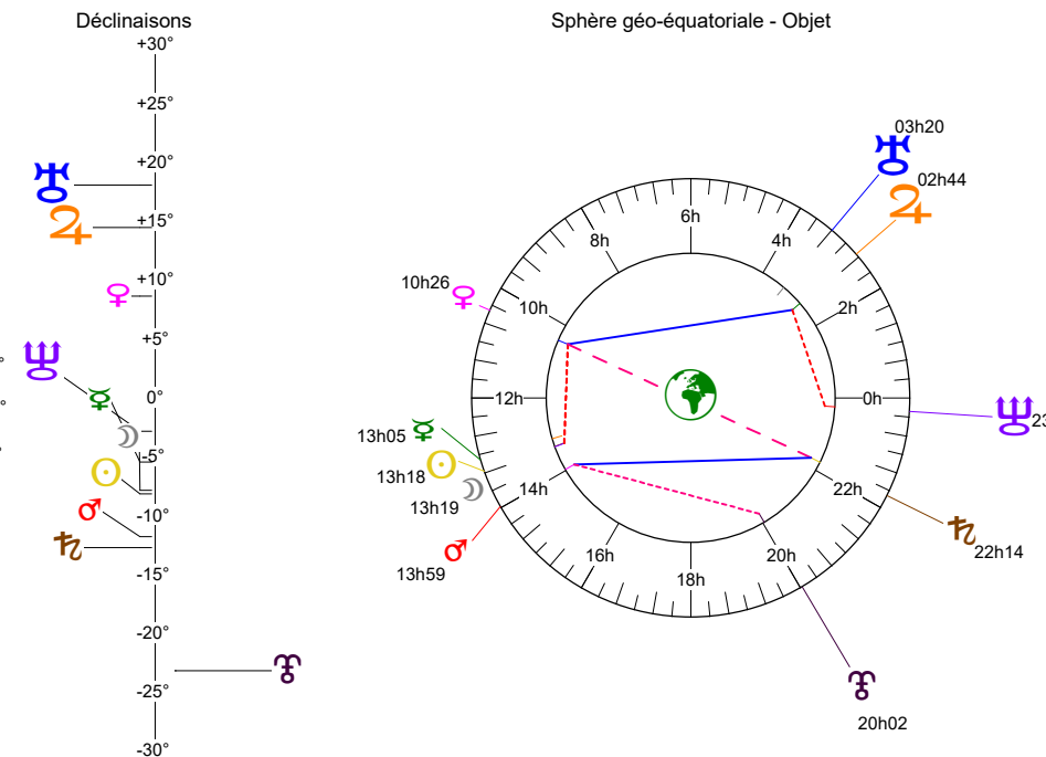
Déclinaisons
