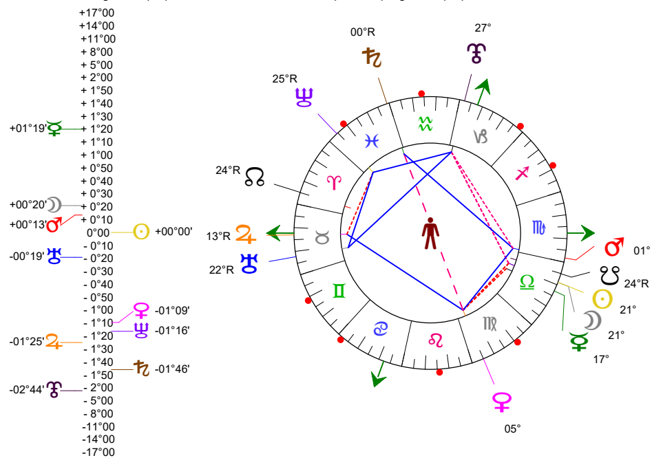
Latitudes géo-écliptiques
