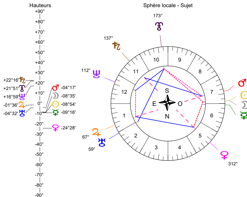
Hauteurs
