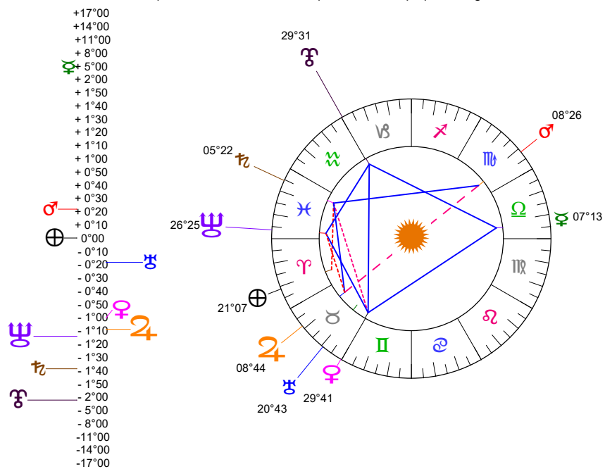
Latitudes héliocentriques
