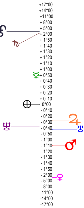
Latitudes héliocentriques
